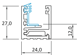
Съставен алуминиев профил
